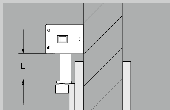
Optionale Wellenverlängerung
