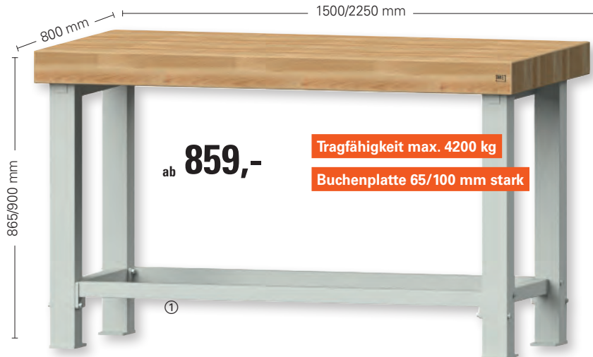
Schwerlast-Werkbank B 1500/2250 x T 800 x H 865/900 mm
