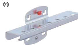
21 Bithalter für 7 Bits H 10 x B 150 x T 35 mm
