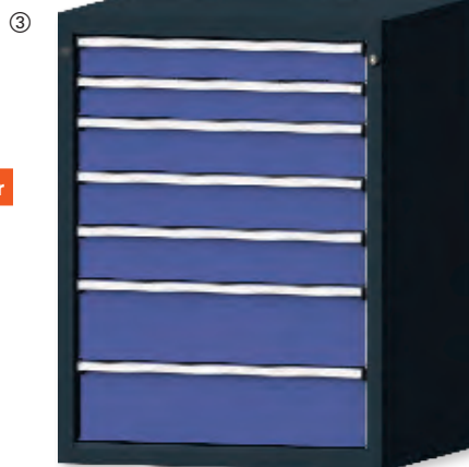
Breite 760 mm, 7 Schubladen 2 x 90, 3 x 120, 2 x 180 mm
