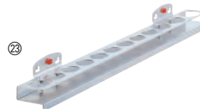
23 Nusshalter für 12 Nüsse H 30 x B 390 x T 45 mm
