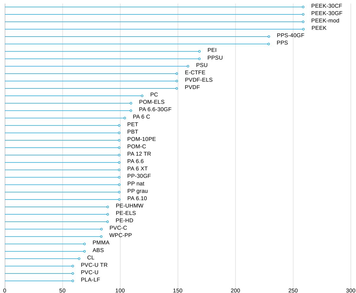
Dauergebrauchstemperatur (°C)
