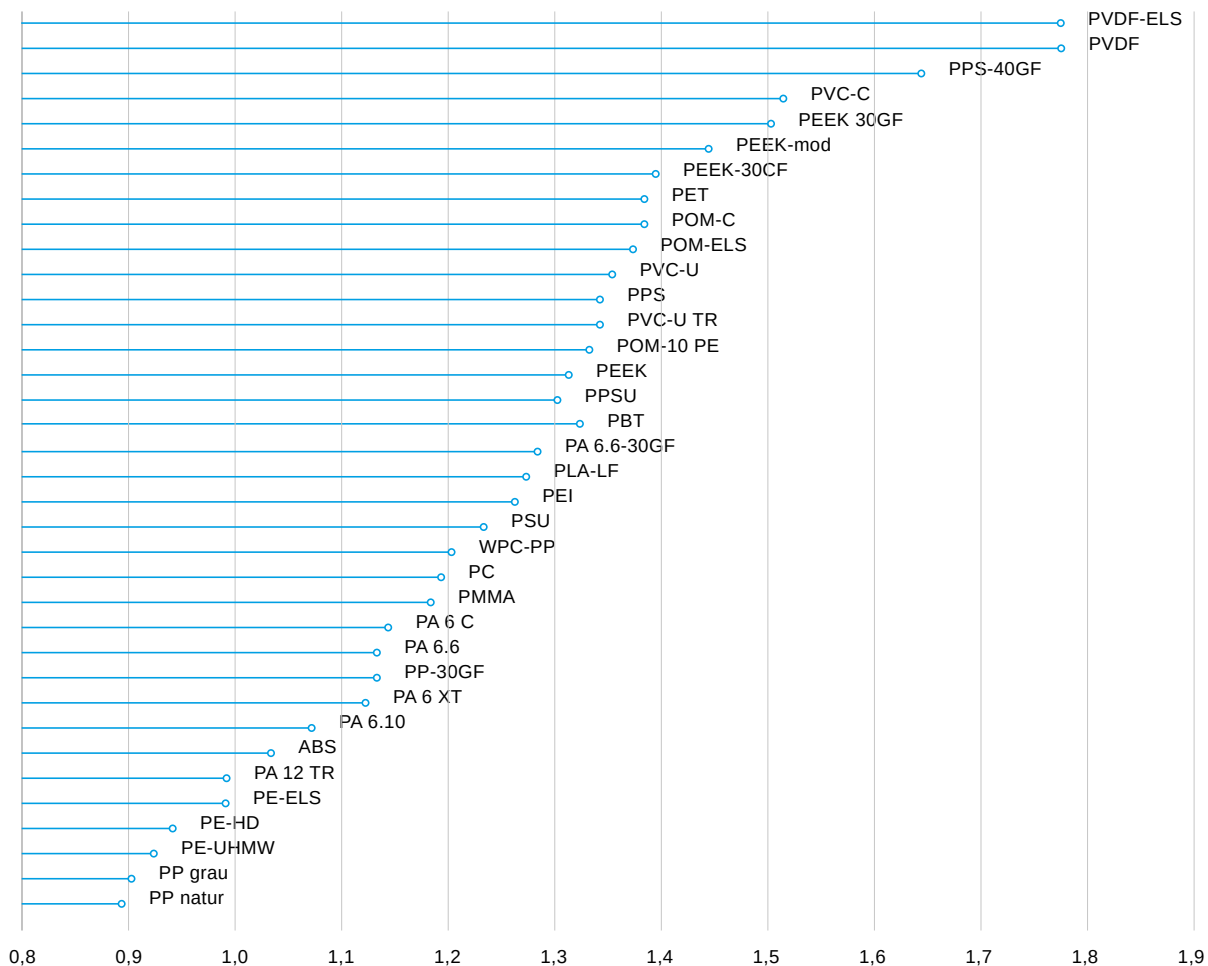
Dichte (g/cm³)
